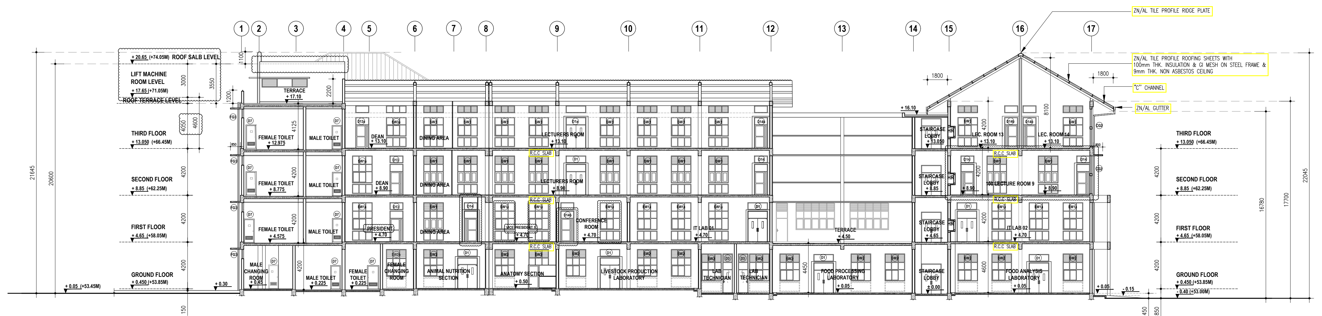
SECTION A-A
