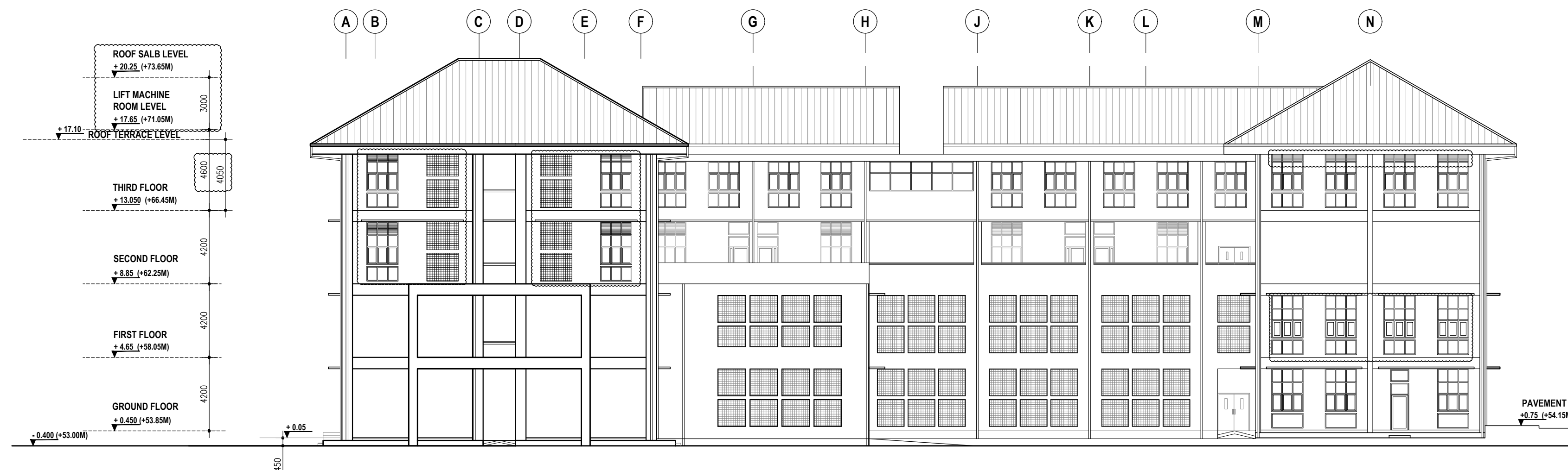
ELEVATION B
